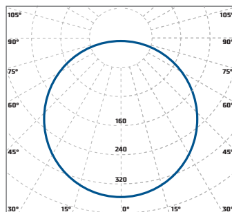
«Diora LPO/LSP Mini opal» косинусная КСС 110°
