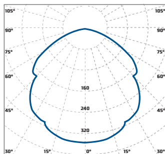
«Diora LPO/LSP Mini» косинусная КСС 120°
